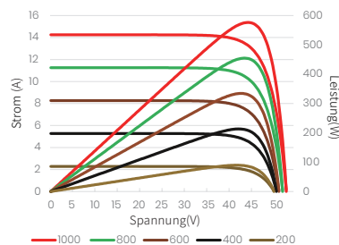
Strom-Spannungs- und Leistungs-Spannungs-Diagramme(585W)
